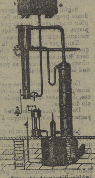
Aparato de rectificación.
