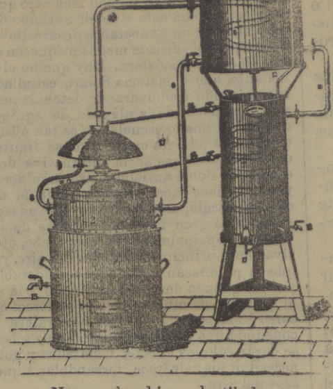
Nuevo alambique destilador.
