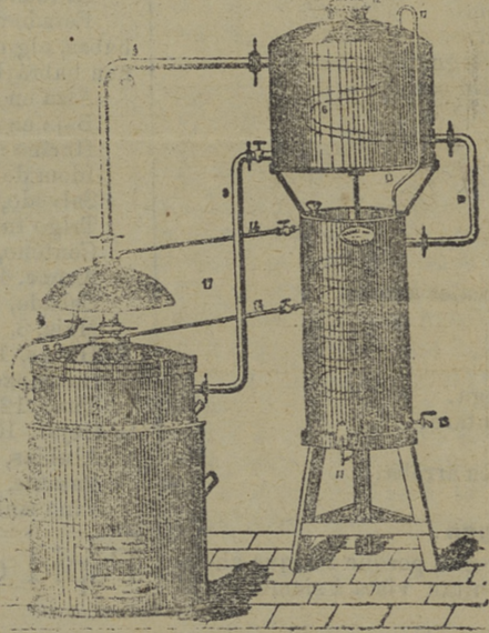
Nuevo alambique destilador.
