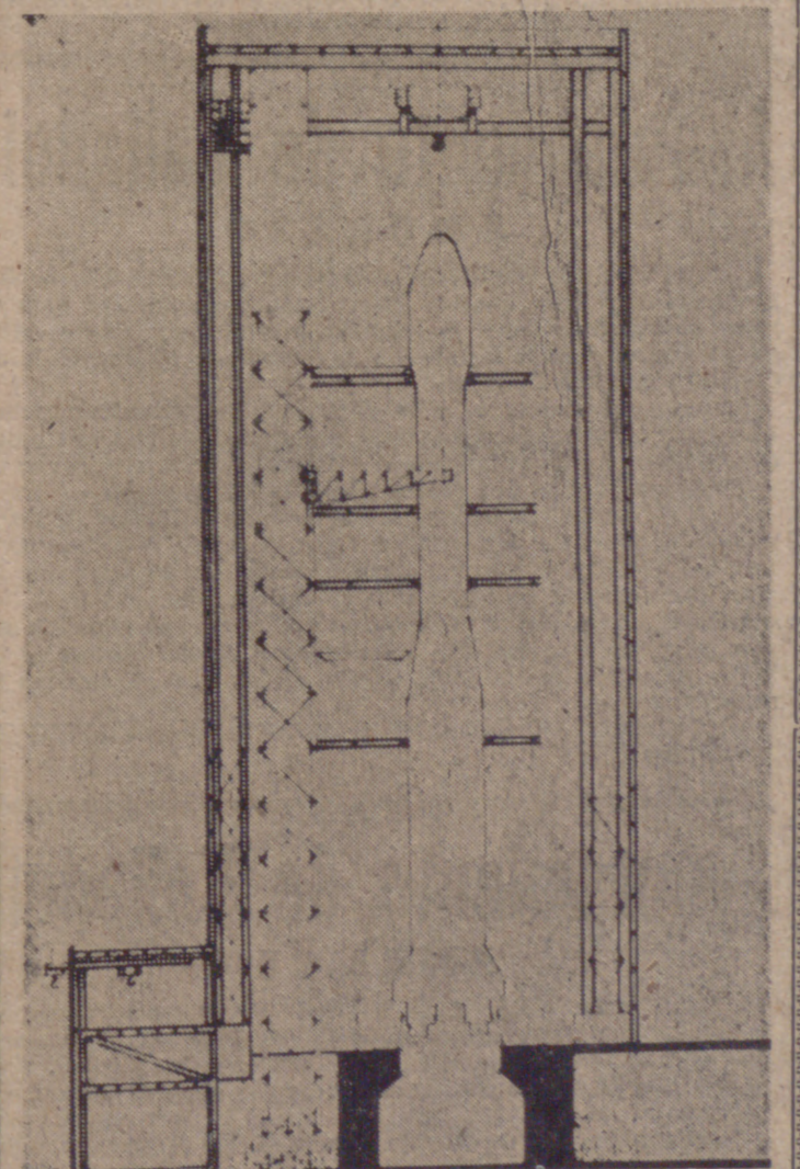
BILBAO.—Gráfico de la torre y plataforma de lanzamiento del cohete del Programa «Ariane» para el lanzamiento de grandes ingenios espaciales. La foto fue facilitada por una empresa vizcaína de ingeniería que participará en la construcción de este cohete.—(Telefoto Cifra Gráfica.)
