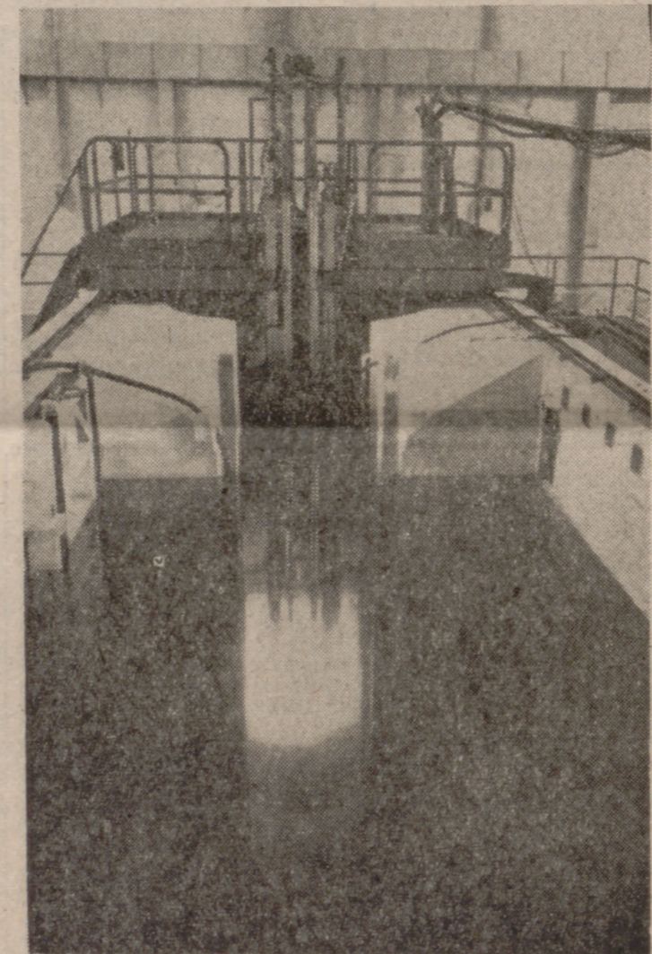
Vista del núcleo del reactor JEN 1.—(Foto PYRESA).
