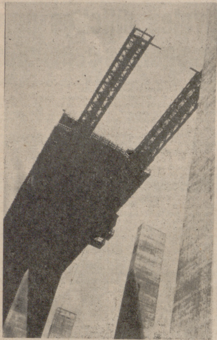
DUSSELDORF.—Nuevos y atrevidos andamiajes facilitan la construcción de puentes sobre valles o sobre ríos. La solución que vemos en la foto se apoya en una cornisa capaz de avanzar de 45 a 50 metros cada quince días.
