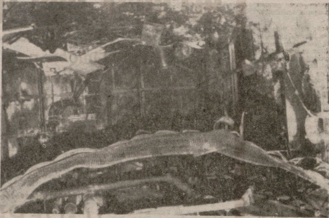
VALENCIA.—Un voraz incendio se produjo a bordo del buque "Rio Neuken", en los astilleros de la Unión Naval de Levante. El buque estaba destinado a una firma armadora argentina e iba a ser entregado en breve plazo. La cuantía de las pérdidas es bastante considerable. En la foto, estado en que quedó una de las bodegas del buque en construcción.—(Telefoto Cifra Gráfica.)
