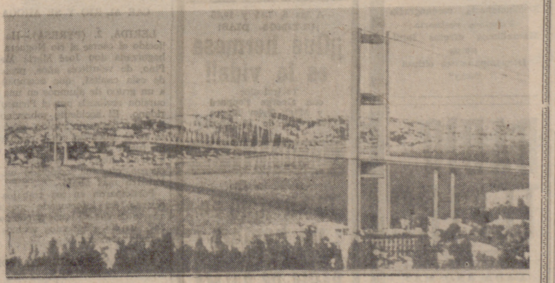
Con una luz de 1.074 metros y una longitud total de 1.560 metros, el puente éurasiático sobre el Bósforo será el más largo de Europa y el cuarto del mundo en cuanto a su longitud (nuestra foto, un montaje con la maqueta). Debajo de sus seis calzadas de 33,40 metros de anchura, colgadas a 64 metros de altura, podrán pasar hasta transatlánticos. Está prevista la terminación de la obra para el año 1973, suponiéndose que atraviesen el puente ya entonces diariamente 22.000 automóviles. Redujo la adjudicación para el proyecto de ciento treinta y cuatro millones de marcos un consorcio germano-ingles. Firmas alemanas, inglesas e italianas suministrarán la estructura metálica.
