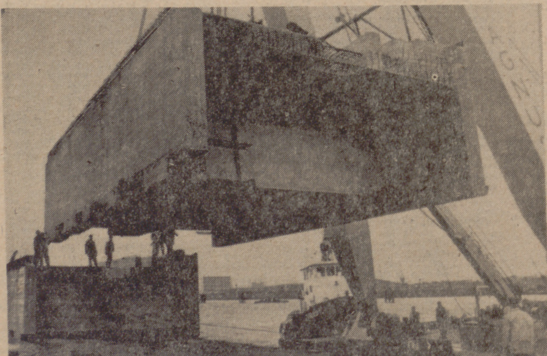
HAMBURGO. (DaD.)—La ampliación del puerto de Hamburgo va progresando rápidamente. En el nuevo muelle, destinado para el amarre de los buques que navegan rumbo Africa están en vías de construcción cinco atracaderos en forma de secciones prefabricadas. En nuestra foto, la grúa flotante "Magnus VII" está colocando un trozo de muro de muelle que pesa 40 toneladas. Para los primeros tres atracaderos del muro, de un total 510 m. de largo, fueron precisas veinticinco de estas secciones de ocho metros de ancho y 3,70 m. de altura. Los gastos de 50 millones de marcos por la nueva instalación, con que quedan sustituidos los viejos tinglados de casi cien años de edad, son repartidos entre la ciudad de Hamburgo y la compañía naviera "Deutsche Afrika-Linien".
