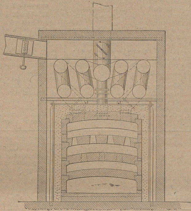
Fig. 2 - Coupe transversale
