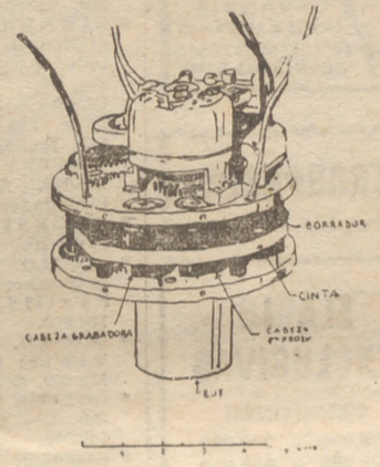
Esquema del sistema telemétrico de un satélite americano. Los datos de los aparatos registradores pasan a los transmisores de radio para ser retransmitidos en forma de señal codificada.
