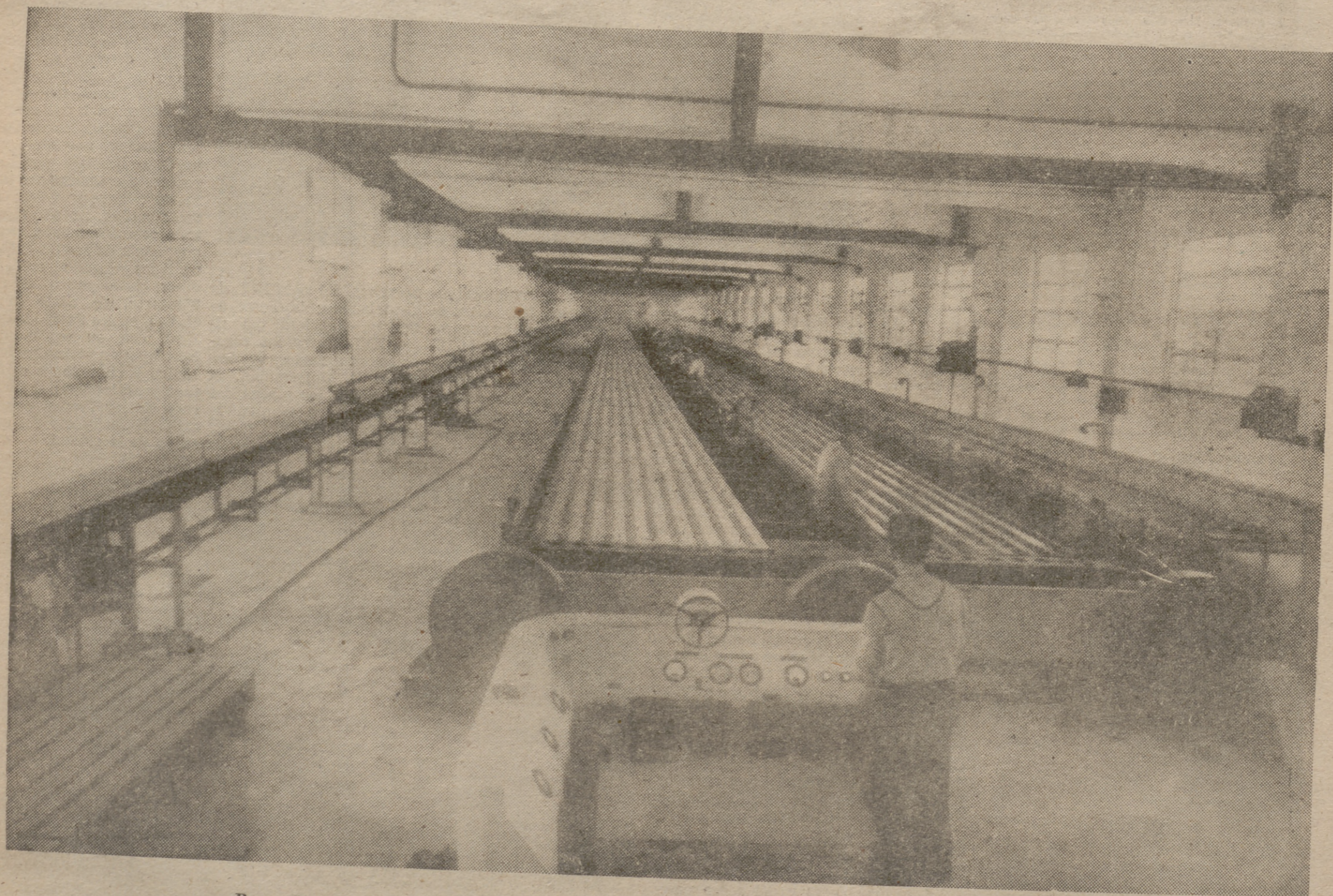
Banco de moldeo múltiple de una de las salas de fabricación de VIGUETAS "CASTILLA", pretensadas.
