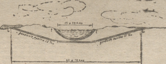
Proyecto del túnel submarino en el Estrecho de Gibraltar
