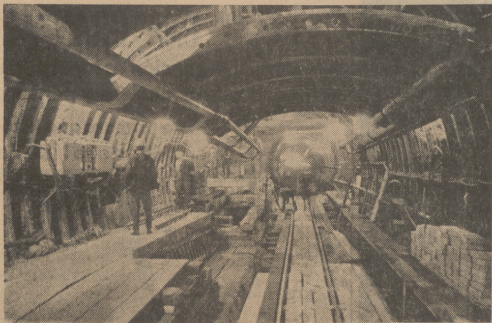
Túnel de la Victoria Line —la línea del Metro londinense de inauguración más reciente—, en construcción. La línea pasa bajo el centro del distrito de tiendas del West End londinense
