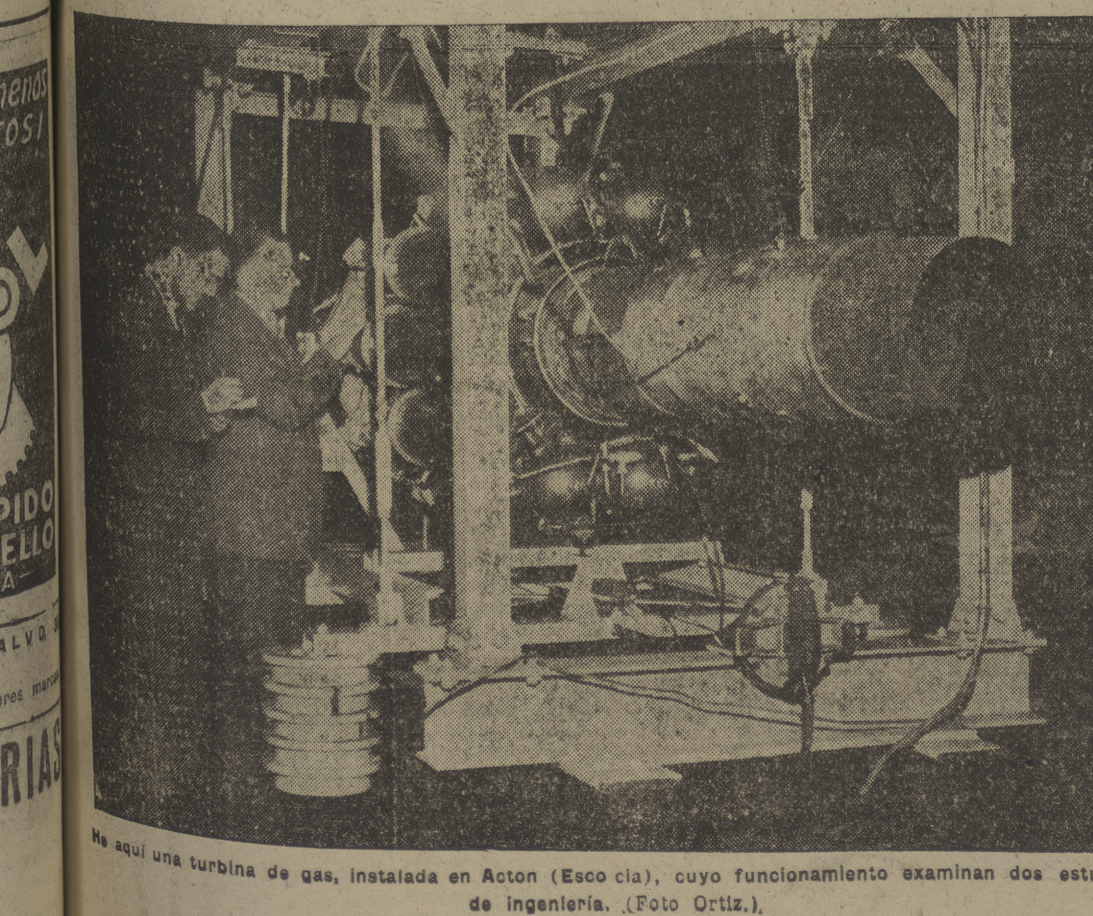
Ma aquí una turbina de gas, instalada en Acton (Esco cia), cuyo funcionamiento examinan dos estudiantes de ingeniería. (Foto Ortiz).
