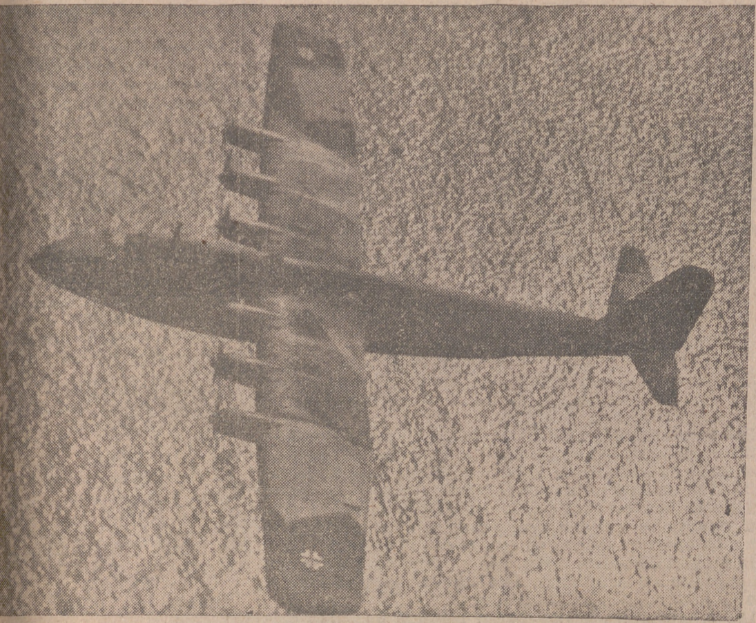
He aquí el hidro «BV 222-Wiking», cuyas características son las siguientes: 37 m. de longitud, 5,6 m. de altura (dos pisos) y 46 m. de envergadura. Este avión ha sido empleado ya con éxito para servicios de los frentes. Su armamento, compuesto de numerosos cañones y ametralladoras, hacen de él una poderosa arma defensiva
