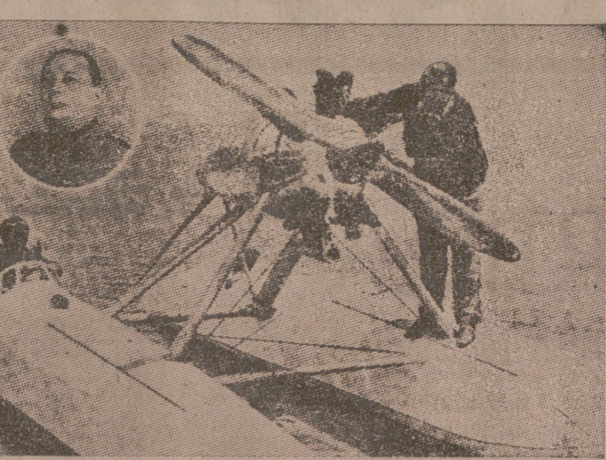
Un nuevo tipo de esquí movido por motor de aviación.—Edgardo Lazzaroni dando el último vistazo a su artefacto antes de comenzar una prueba
