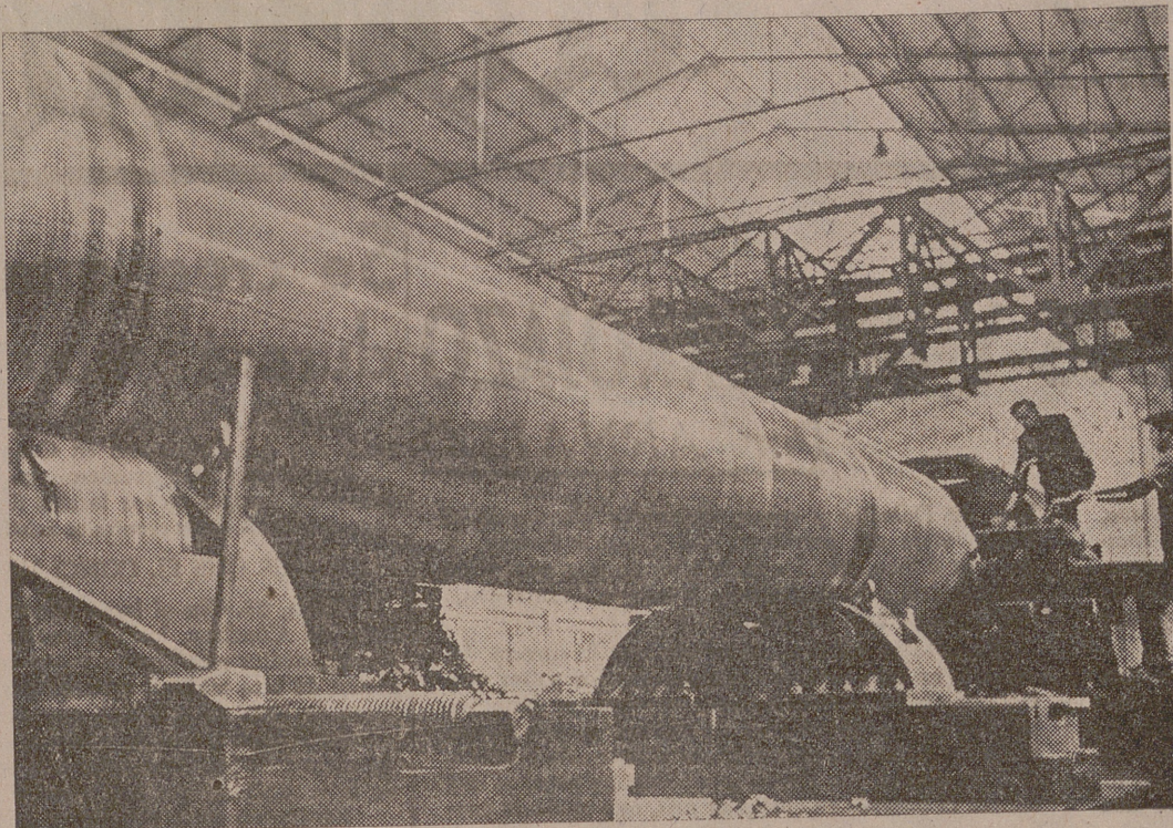
Una fotografía de los grandes establecimientos "Unión de minas Dortmund-Hoerder" (Alemania). Parte de la maquinaria necesaria para obtener gasolina del carbón
