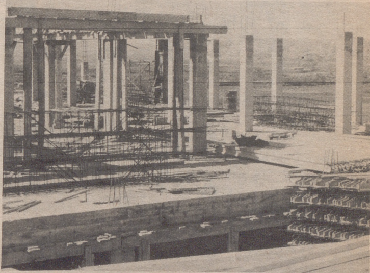
Estado actual de las obras. Al fondo, el valle del Jiloca (Foto del autor)
