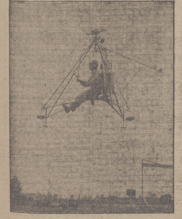
El primer helicóptero de propulsión a chorro de la Marina norteamericana, el RH-1, se eleva en el aire en unas pruebas efectuadas en la base aérea de los Alamitos (California). Se ha tardado cerca de cuatro años en diseñar este monoplaza. Sus características le hacen recomendable para las operaciones de reconocimiento y observación. Una de las novedades de este helicóptero es el control del motor por medio de una válvula. Los modelos anteriores sólo disponen de «encendido» y «apagado».
