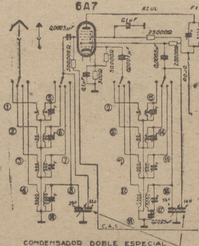
Fig. 159.—Circuito "Banda ensanchada".
