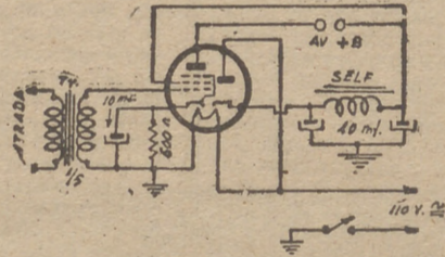
Fig. 158. Amplificador de baja frecuencia para aparatos de galena.
