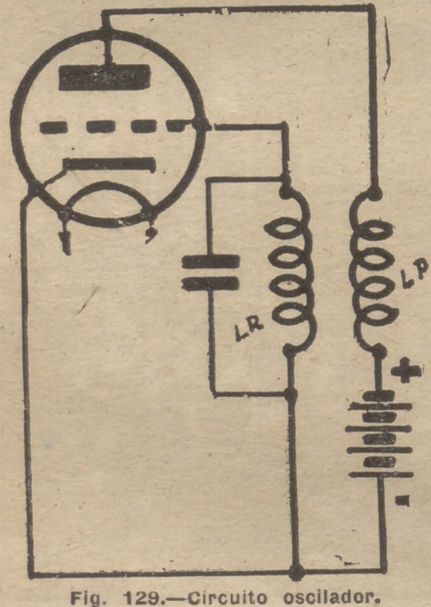
Fig. 129.—Circuito oscilador.
