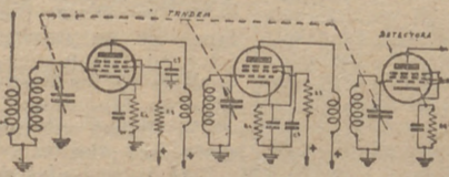
Fig. 123. — Circuito "radiofrecuencia sintonizada".
