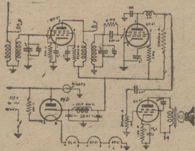
Fig. 124.—Esquema de un receptor universal tipo de amplificación directa (R. F. S.)
