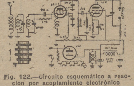
Fig. 122.—Circuito esquemático a reacción por acoplamiento electrónico
