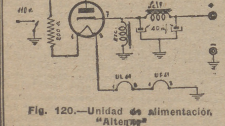
Fig. 120.—Unidad de alimentación "Altern"
