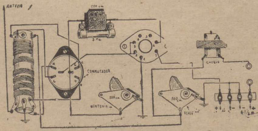
Fig. 112.—Conexión práctico del circuito de la figura 111
