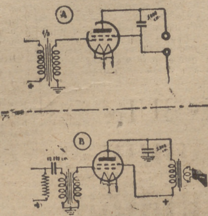
Fig. 113.—Variantes del circuito amplificador de baja frecuencia
