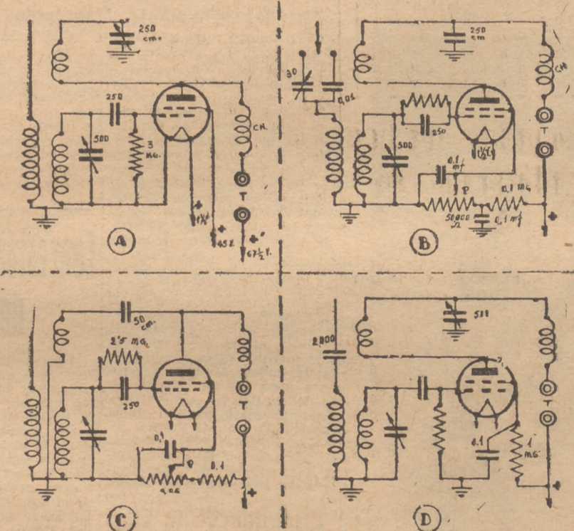
Fig. 110.—Variantes del circuito de una lámpara detectora a reacción
