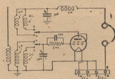
Fig. 111.—Circuito detector a reacción que emplea dos longitudes de ondas
