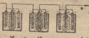
Fig. 55.—Montaje de pilas en serie.
