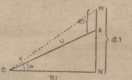
Triángulo de tensiones en circuito con reactancia y con capacitancia
