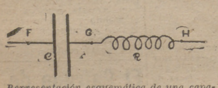
Representación esquemática de una capacidad en serie con una reactancia
