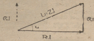
Triángulo de tensiones
