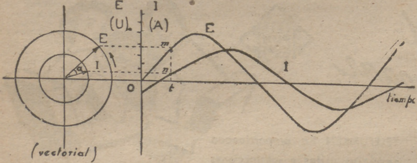
Corriente alterna en un circuito inductivo
