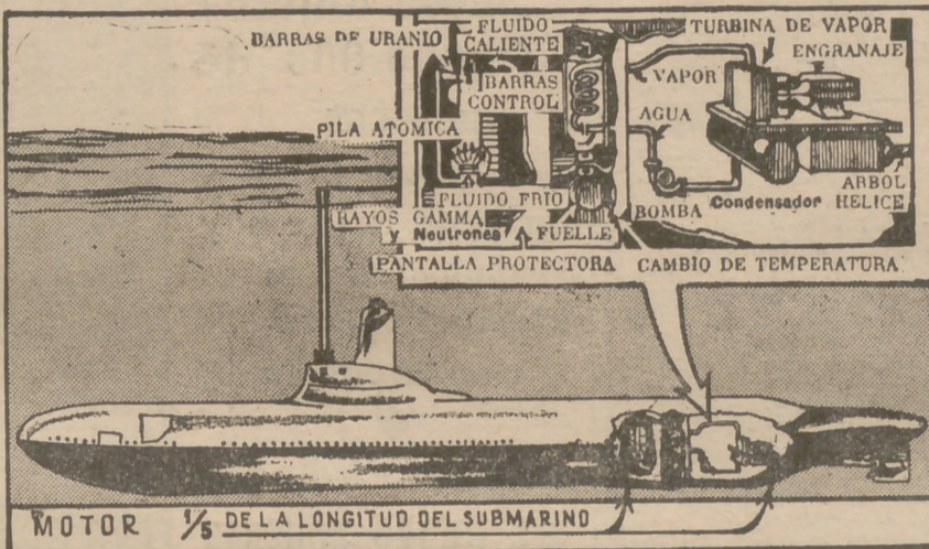
MOTOR 1/5 DE LA LONGITUD DEL SUBMARINO
