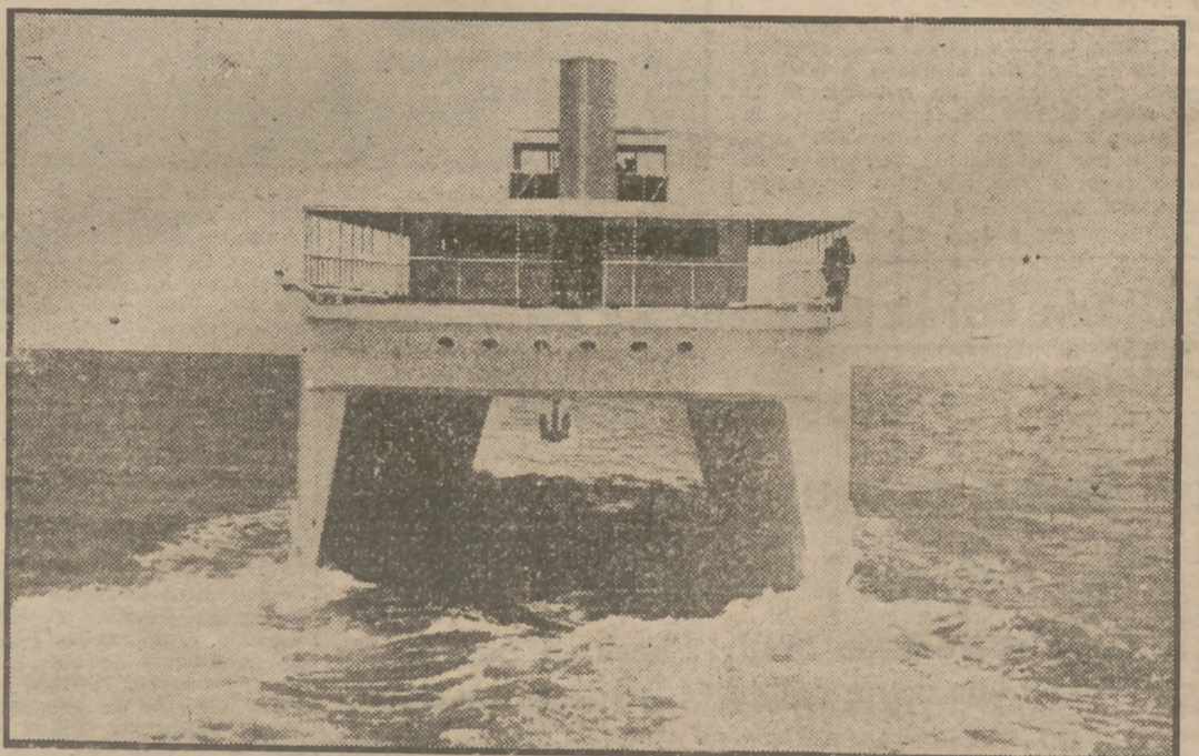
Este es el "Venturi", buque del nuevo modelo que ha inventado Gar Wood, cuya característica más saliente es la de tener dos quillas, lo que le da más estabilidad sobre el mar, a la vez que le permite mayores velocidades, por su menor resistencia. (Foto A. P.)
