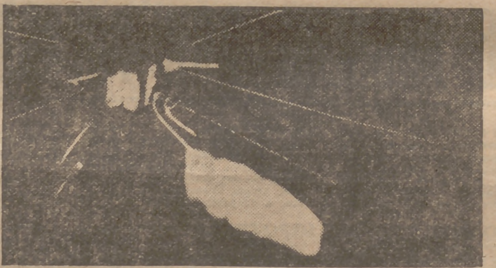
Fotografía tomada en "cámara de nubes" del momento de la desintegración de un átomo bombardeado con protones.
