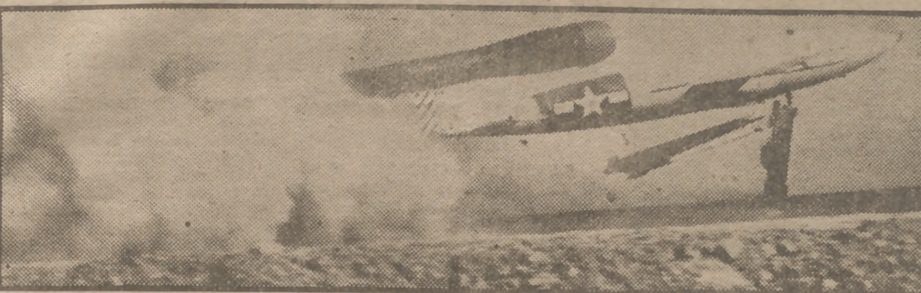
Por ingenieros navales norteamericanos ha sido construida y probada esta bomba-cohete, en la que se han mejorado los principios de la V-1 alemana. El nuevo proyectil, conocido por la KUW-1, alcanza una velocidad de 425 millas hora y su radio de acción es de 150 millas. Al producirse el lanzamiento se desprende el mecanismo que lo produce. (Foto Philips.)
