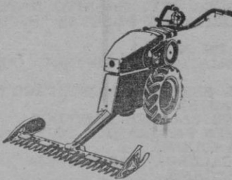
motosegadora barra de corte 1,10 mts. 3 marchas adelante y 1 atrás
