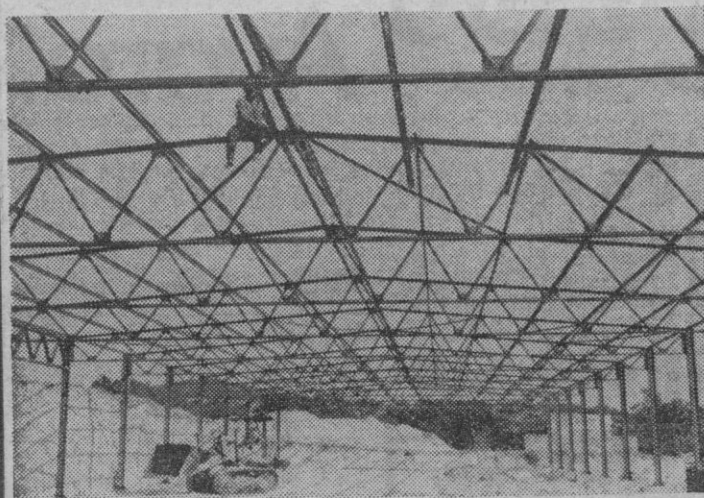
ESTRUCTURA METÁLICA PARA «VIBRADOS Y PRETENSADOS». - MANACOR. - 2.ª NAVE, DE 20 x 100 METROS.
