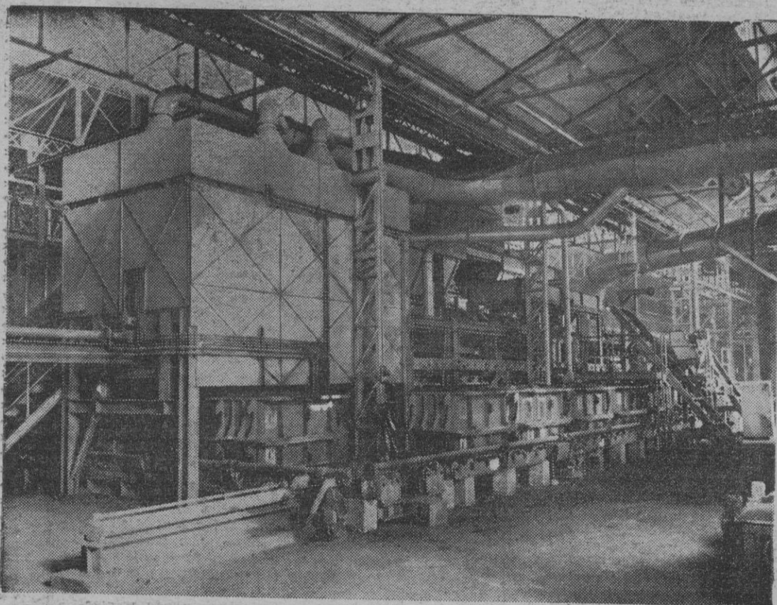
VISTA PARCIAL DE LA MAS MODERNA FACTORIA AUTOMATICA DE BANERAS DE HIERRO FUNDIDO DEL MUNDO, CON CAPACIDAD PARA PRODUCIR UNA BANERA CADA 49 SEGUNDOS
