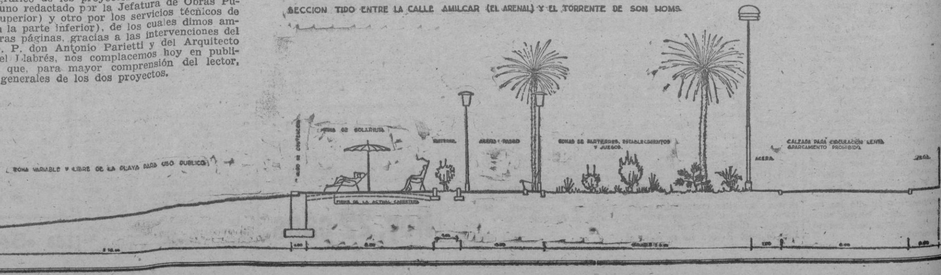
SECCION TIDO ENTRE LA CALLE AMILCAR (EL ARENAL) Y EL TORRENTE DE SON MONS.
