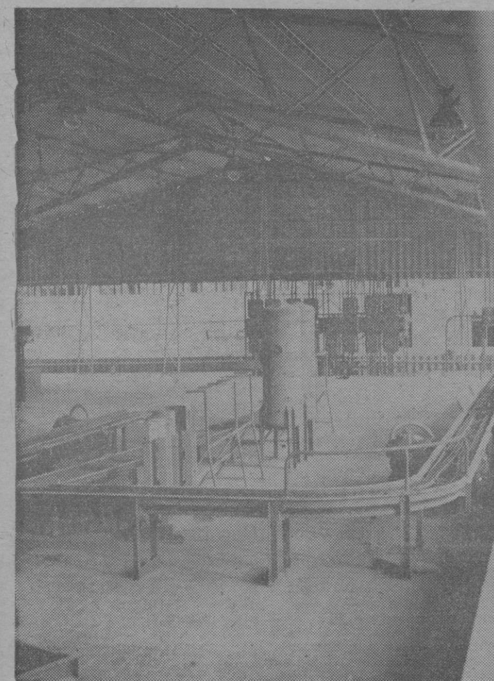
BUTANO S. A. PLANTA ENVAÑADO GAS. PUERTO ALCUDIA. (EN MONTAJE)
