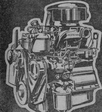
Modelo 4/99 V - 11-HP fiscales 44 HP a 4.000 r. p. m.
