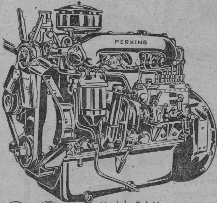
Modelo P 6 V 26 HP fiscales 84 HP a 2.400 r. p. m. 89 HP a 3.000 r. p. m.
