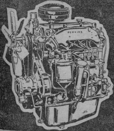
Modelo P 4 V - 17 HP fiscales 63 HP al freno
