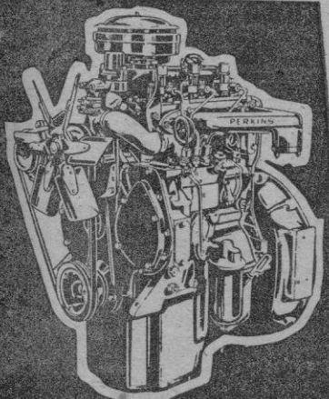
Modelo P 3 V - 13 HP fiscales 41 HP al freno
