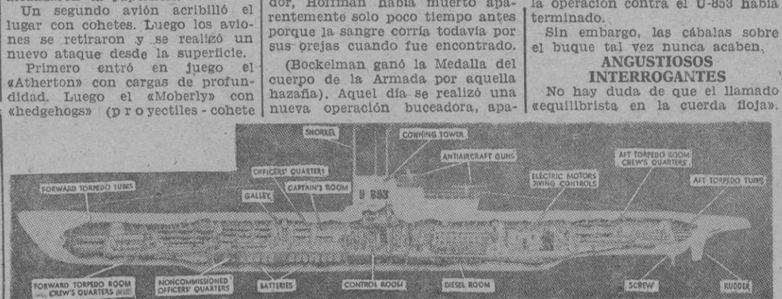
He aquí un corte ideal del submarino alemán U-853. El navío era uno de los más perfeccionados que fueron puestas al servicio por la Marina alemana. Estaba equipado con un «snorkel», mecanismo que permite a los motores Diesel «respirar» debajo del agua y prolongar grandemente las inmersiones del buque. — (FOTOFIEL).
