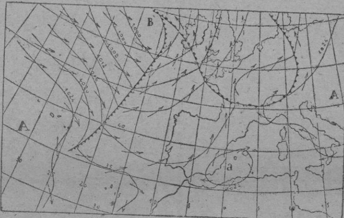
Mapa sinóptico correspondiente al día de ayer, 21-1-61 a 07 horas Z (08 oficiales). — Las líneas finas representan isobaras; y los números son presiones en milibares (1.000 milibares: 750 mm. de mercurio). Las letras A y B designan respectivamente centros anticiclónicos y depresionarios. La línea festoneada es el frente. Las flechas señalan la dirección del viento.
