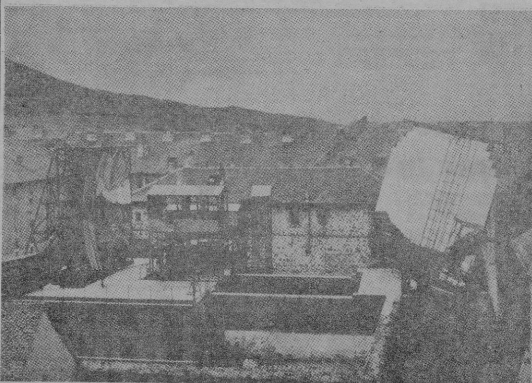
En la antigua fortaleza de Mont-Louis, en los Pirineos, un espejo plano (derecha) sigue el paso del sol a través del cielo y refleja sus rayos sobre un espejo parabólico (izquierda) que los concentra en el orificio de un horno solar, al centro. — (Foto Laboratorio de energía solar de Mont-Louis.)
