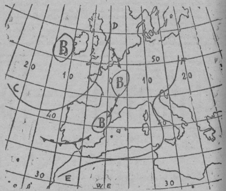
Situación del Tiempo el sábado día 14 por la mañana. La línea CD señala el límite de la extensa depresión del Atlántico que tiene su centro al oeste de Irlanda. La línea EF representa el límite de la presión normal; a la izquierda es algo más baja, con dos pequeños centros (B B) ensartados a lo largo de un frente estacionario.
