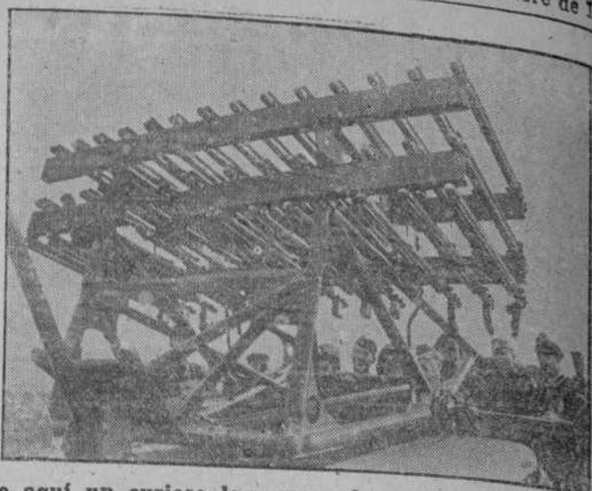
He aquí un curioso lanzagranadas soviético encontrado por las tropas alemanas en uno de los numerosos botines cogidos. Es automático y pueden dispararse 42 granadas a la vez.
