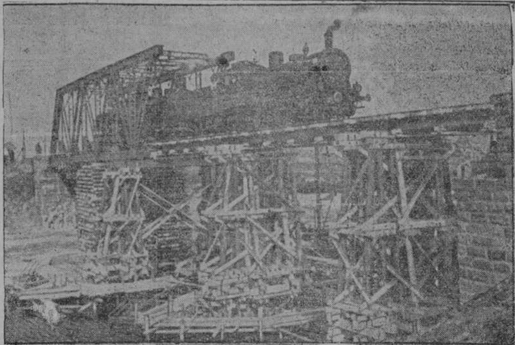
Para probar la resistencia de un puente construido por los pontoneros alemanes en Rusia, se hacen pasar por él dos locomotoras pesadas.
