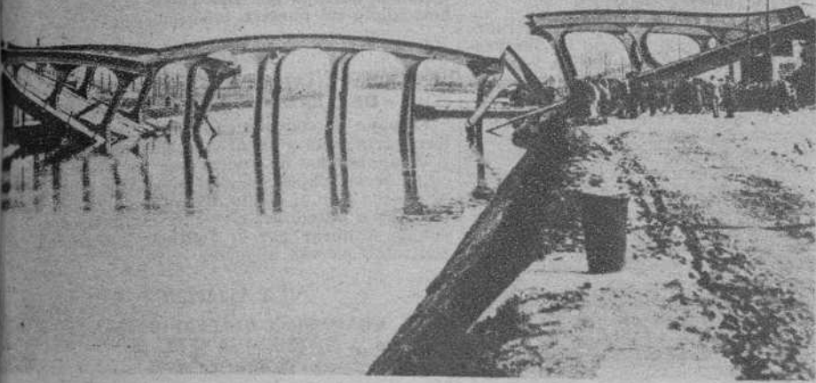
HUNDIMIENTO DE UN PUNTE EN BELGICA. — Inmediatamente después de haber pasado un tren con muchísimos pasajeros sobre el gran y nuevo puente del estratégico de Alberto, en Hasselt, se hundió. Ingenieros militares acudieron en seguida al lugar siniestro, para construir un puente provisional, por ser éste de suma importancia. El puente fue construido hace un año, con material alemán, y se encuentra a 16 millas de Eindhoven. Aunque no se haya encontrado todavía una huella definitiva, se supone que el hundimiento es debido a un acto de sabotaje.
