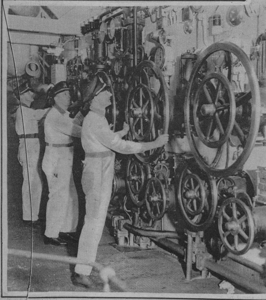
El cuarto de máquinas del «Leviathan», el mayor buque de pasajeros de los E.E. U.U.
