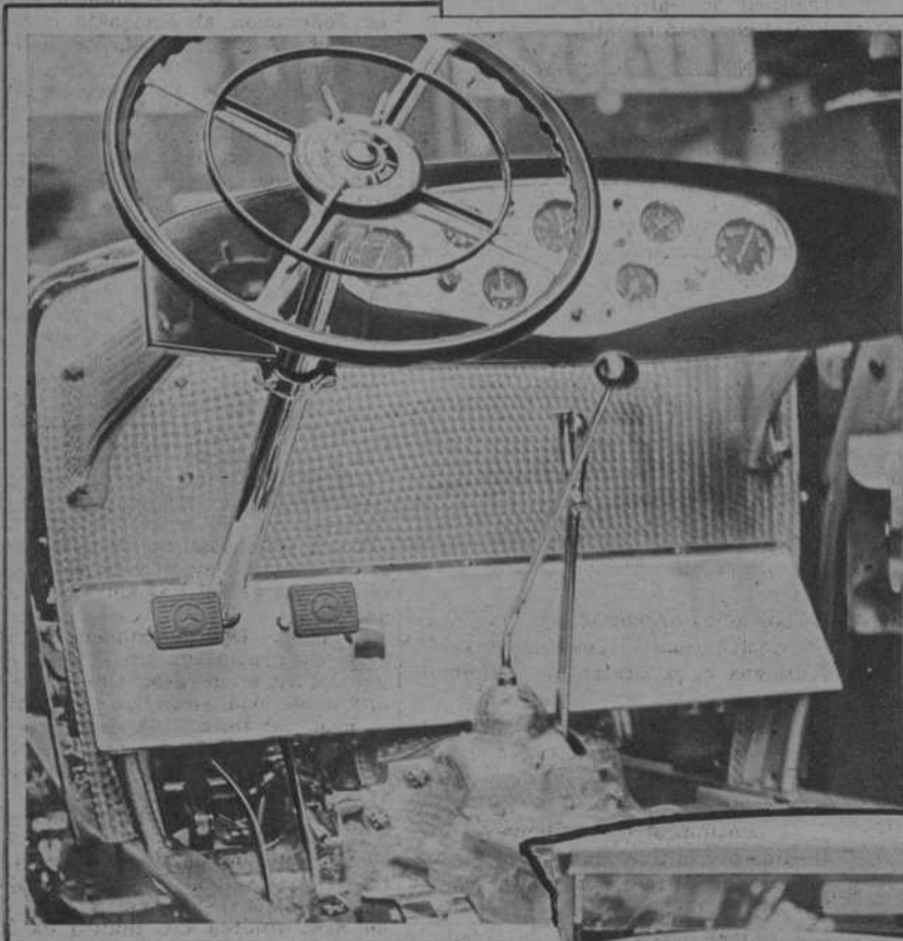
Un detalle de la nueva técnica de un modelo expuesto en el «Salón»
