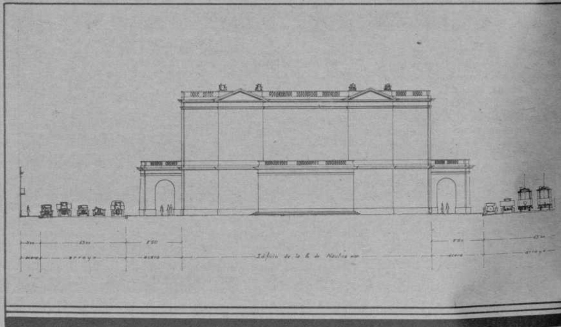
Corte vertical que da idea del espacio que queda libre para el tránsito público
