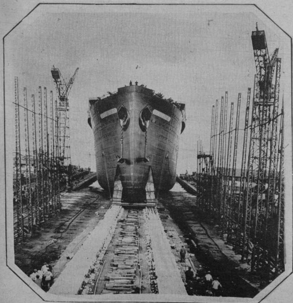
El trasatlántico francés «L'Atlantique», de 39.000 toneladas, que acaba de ser botado al agua con toda felicidad
